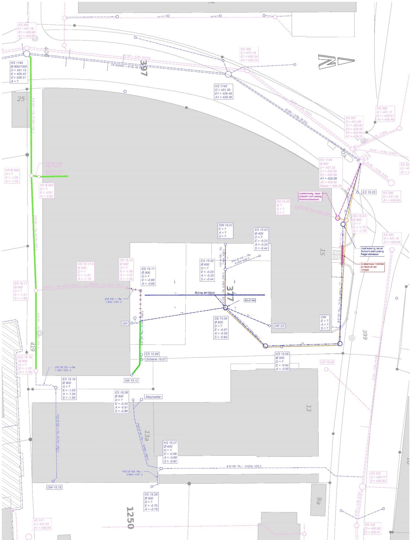
Situationsplan Vorprojekt
